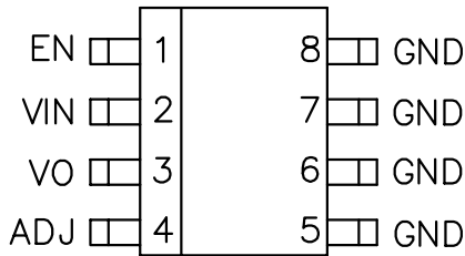
SO-8
